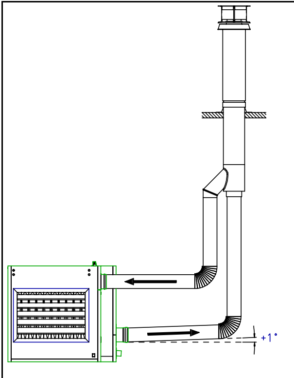
Figuur 11b : VERTIKALE AAN- & AFVOER
