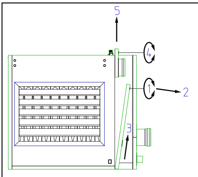
Figuur 17 : TOEGANG TOT BRANDER
