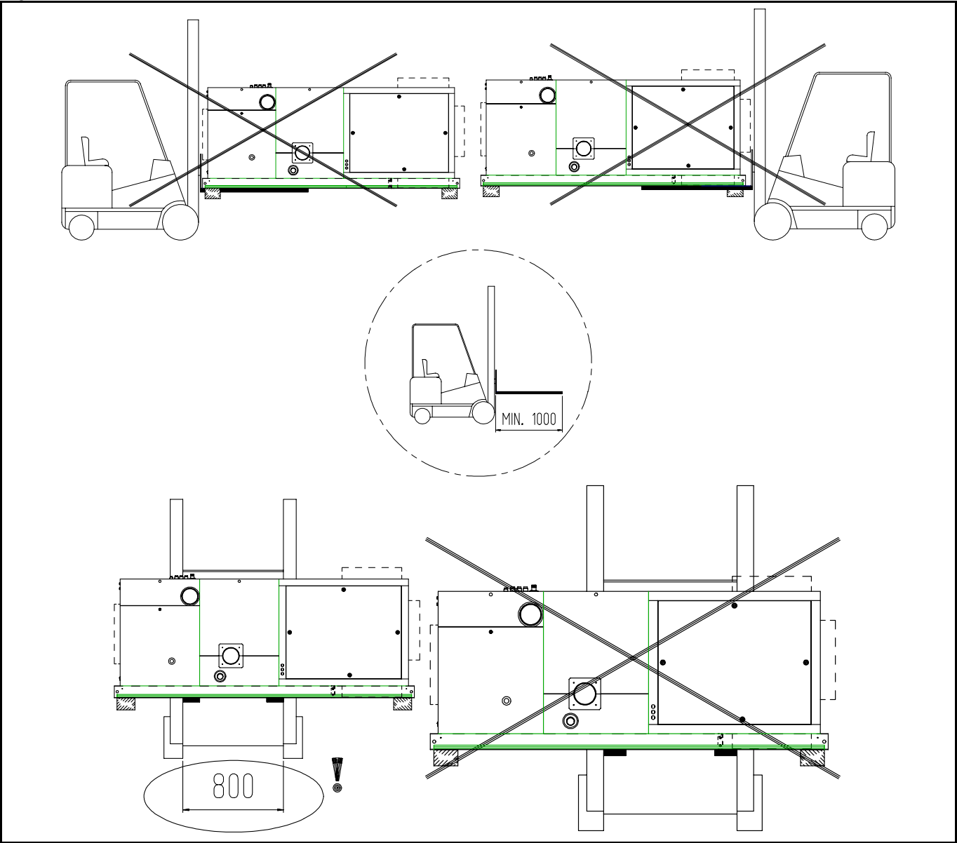
Figuur 2 : TRANSPORT & OPTILLEN TOESTEL
