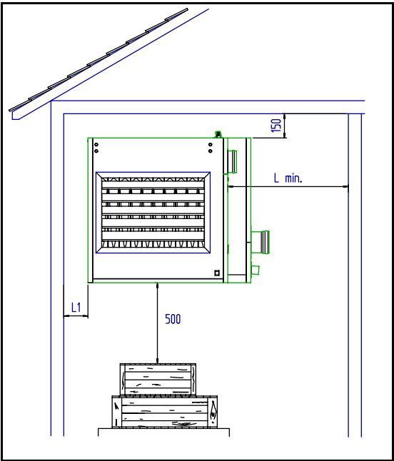
Figuur 3 : AFSTANDEN EN MONTAGE
