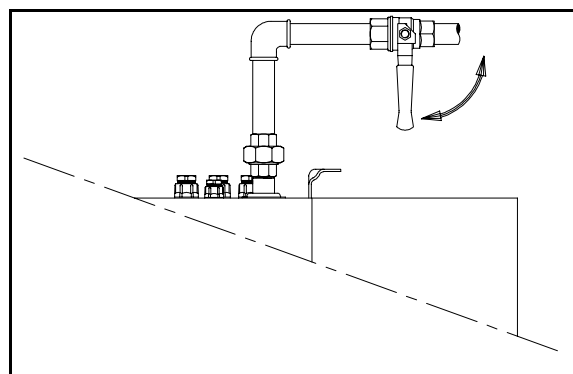
Figuur 14 : DETAIL GASAANSLUITING
