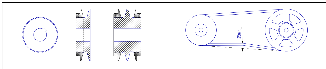
Figuur 15 : INSTELLEN VENTILATORSNELHEID
