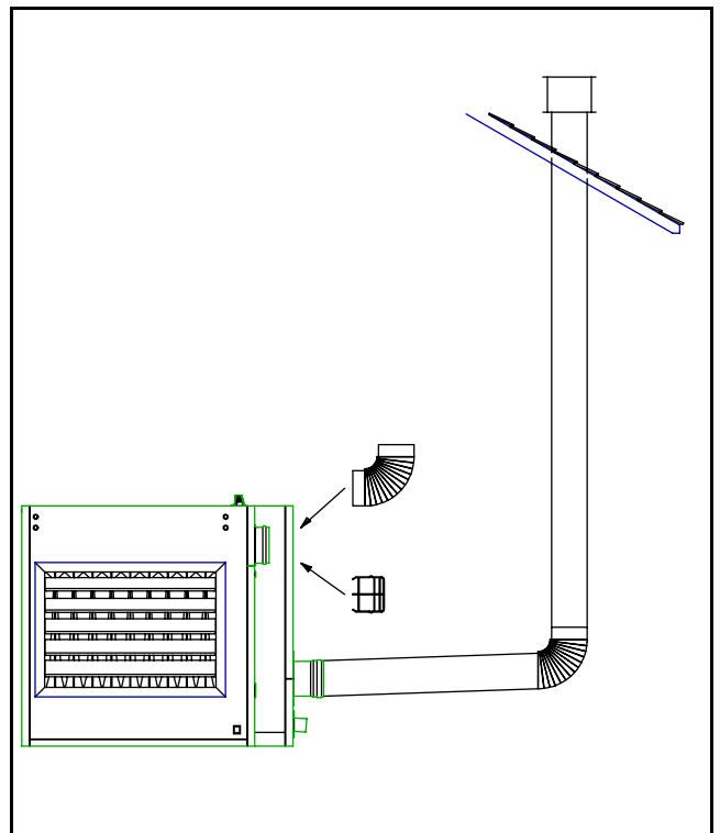
Figuur 12 : TYPE B TOESTEL
