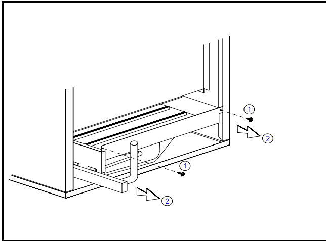
Figuur 20 : VERWIJDEREN BRANDERREK
